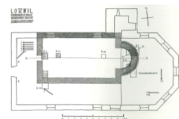
Grundriss der Kirche über dem Fundament der früheren Kirche.
